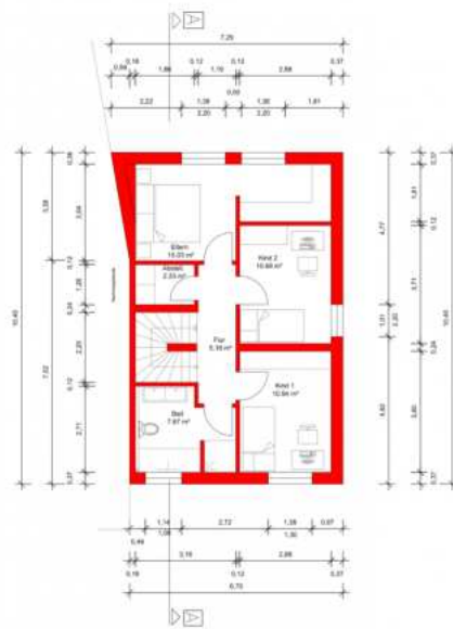
OG_Grundriss
